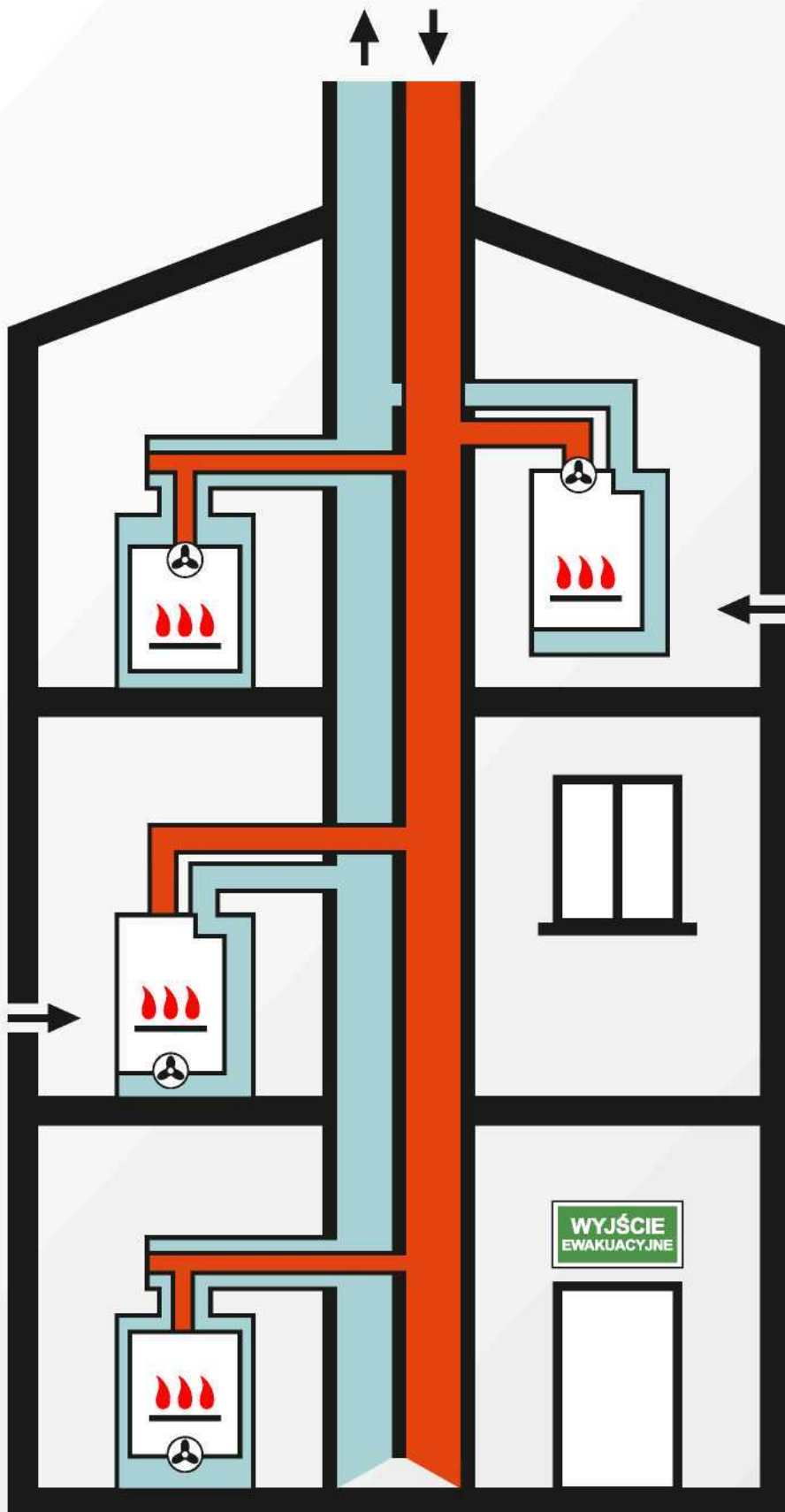
Przykład konfiguracji systemów kominowych i wentylacyjnych (dla kotłów opalanych gazem typu C4)
